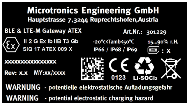
Typenschild
