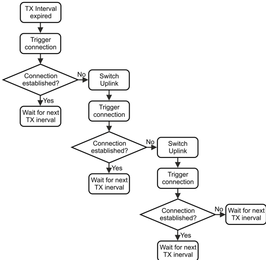
Ablauf der automatischen Umschaltung der Mobilfunktechnologien
