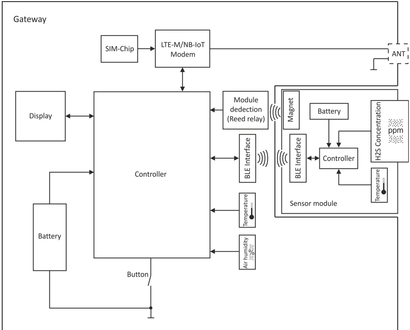
Blockschaftbild des myDatasensH2S1000 LTE-M
