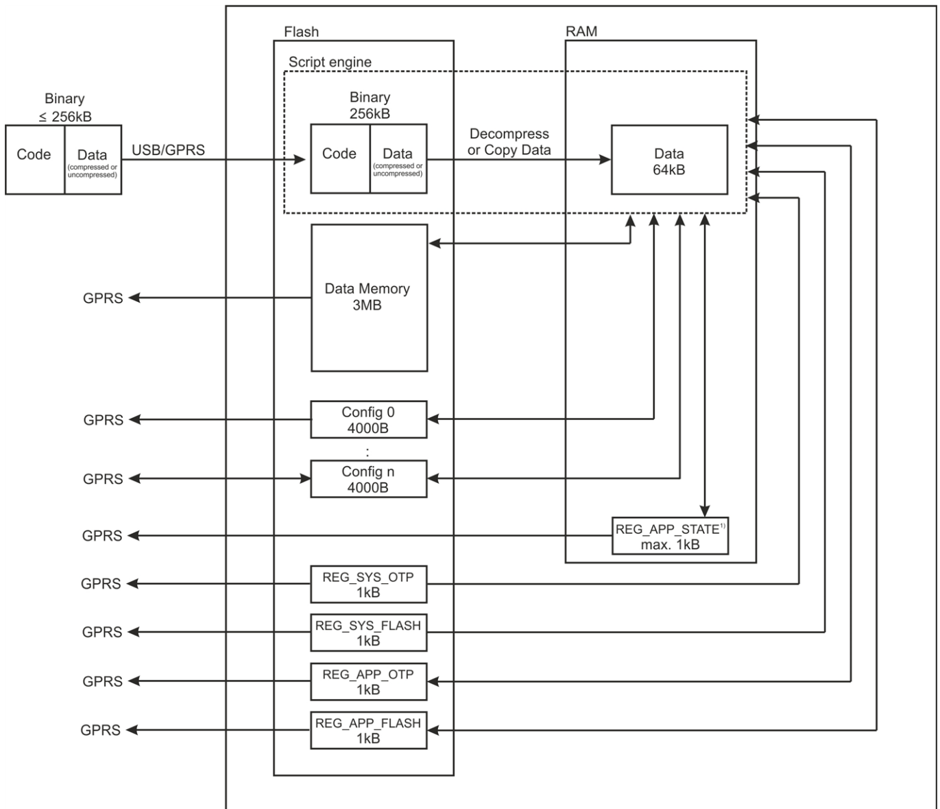
Organisation des Speichers des myDatalogC32x
