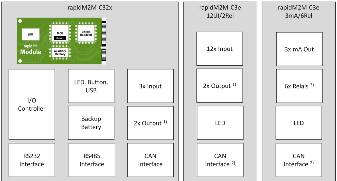
Systemarchitektur des myDatalogC32x und der Erweiterungsmodule
