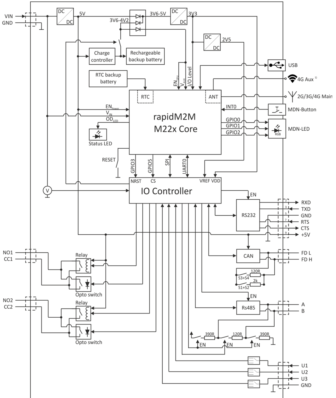
Blockschaltbild des myDatalogC32x
